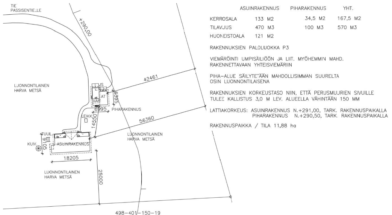
Kuva 14. Ote suunnittelutarveratkaisun asemapiirroksista. © Insinööritoimisto Reino Niemitalo Oy.
